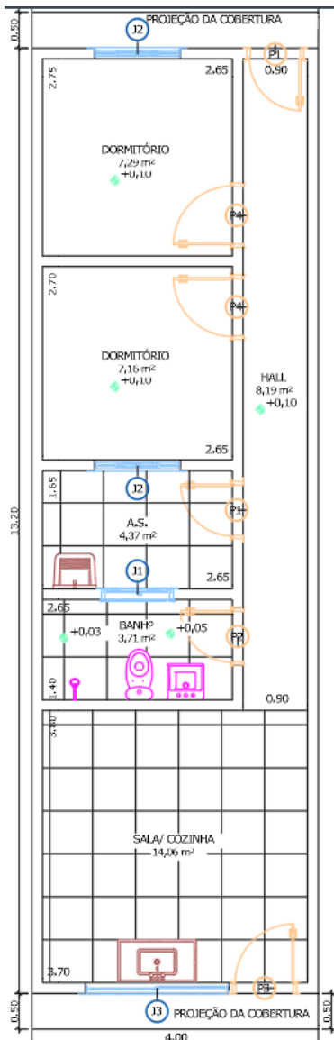
PLANTA BAIXA SEM ESCALA
