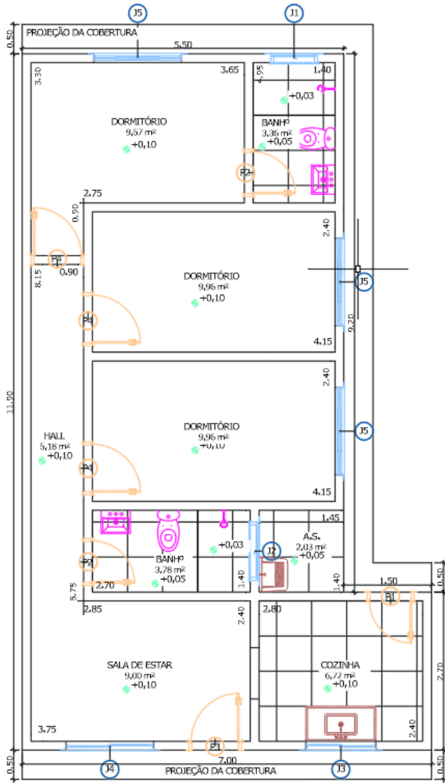
PLANTA BAIXA SEM ESCALA
