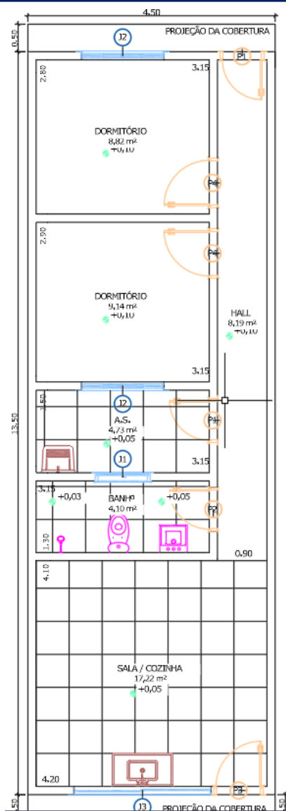
PLANTA BAIXA SEM ESCALA
