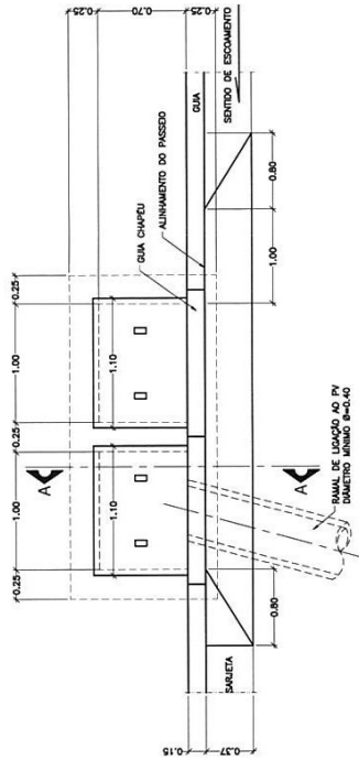
PLANTA-Boca de lobo dupla OBSERVAÇÕES 1, 2, 3, 4 e 5
