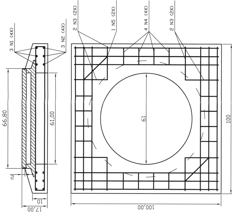
ARMAÇÃO DA LAJE unidade = cm
