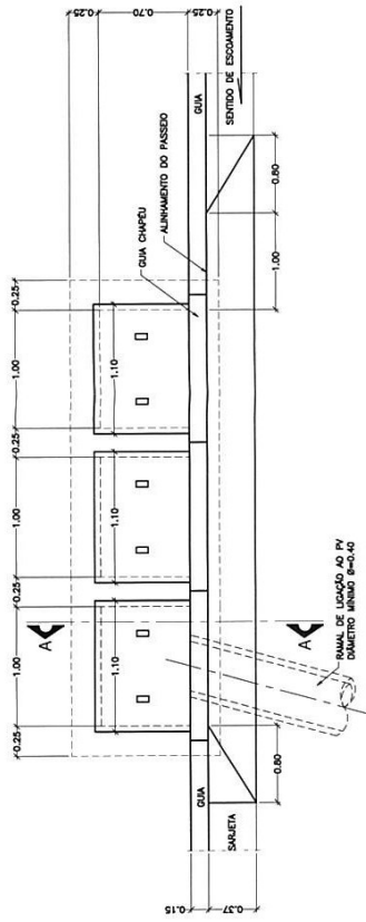
PLANTA-Boca de lobo tripla OBSERVAÇÕES 1, 2, 3, 4 e 5
