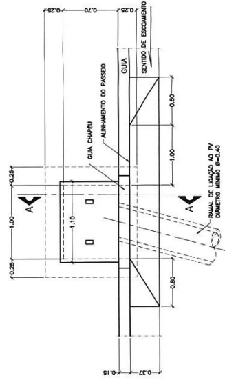
PLANTA-Boca de lobo simples OBSERVAÇÕES 1, 2, 3, 4 e 5
