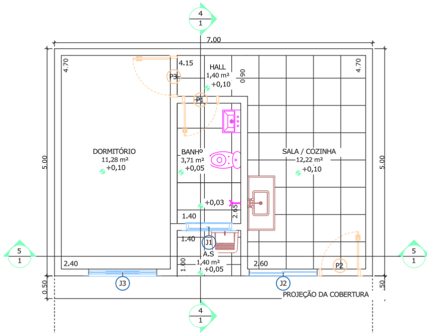
PLANTA BAIXA SEM ESCALA
