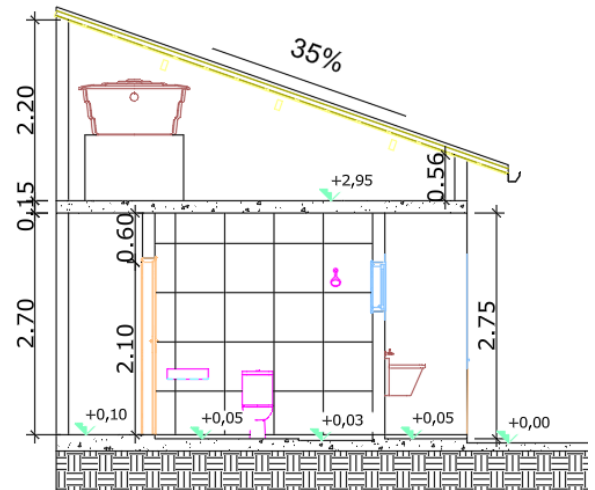
CORTE SEM ESCALA
