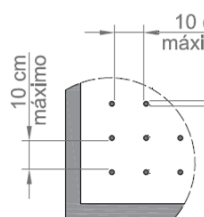
Detalhe A ex. adesivo circ
