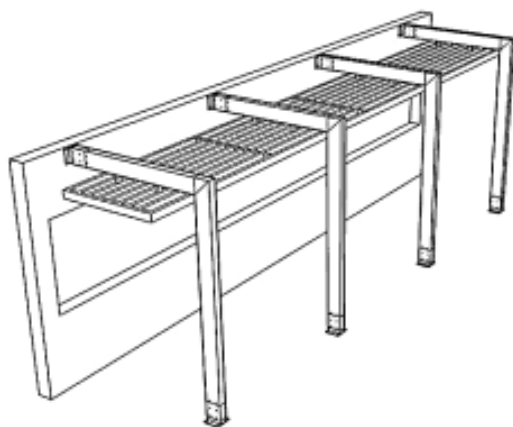
Figura 31. Sombreador externo horizontal com aletas.
