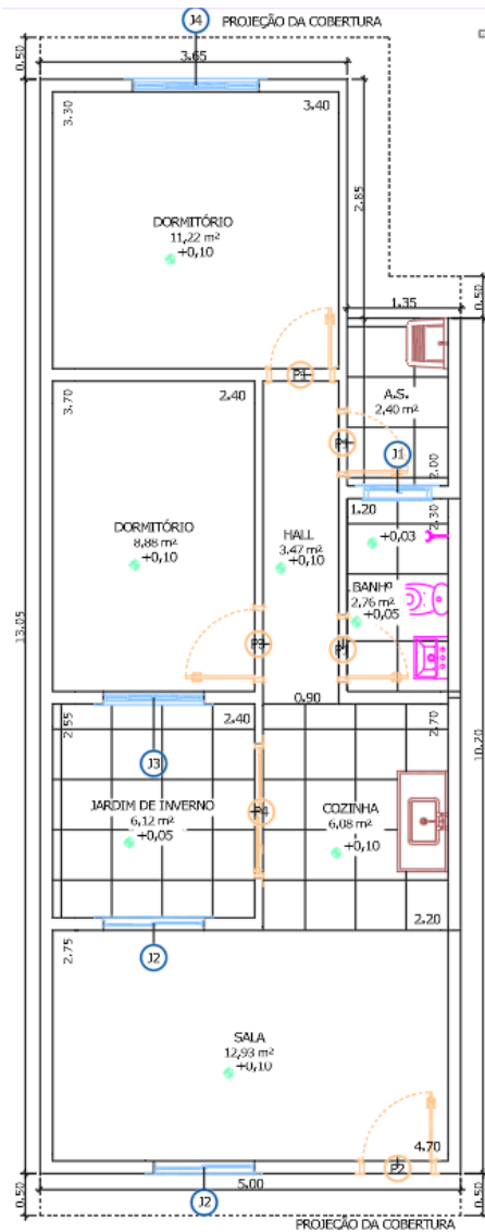
PLANTA BAIXA SEM ESCALA
