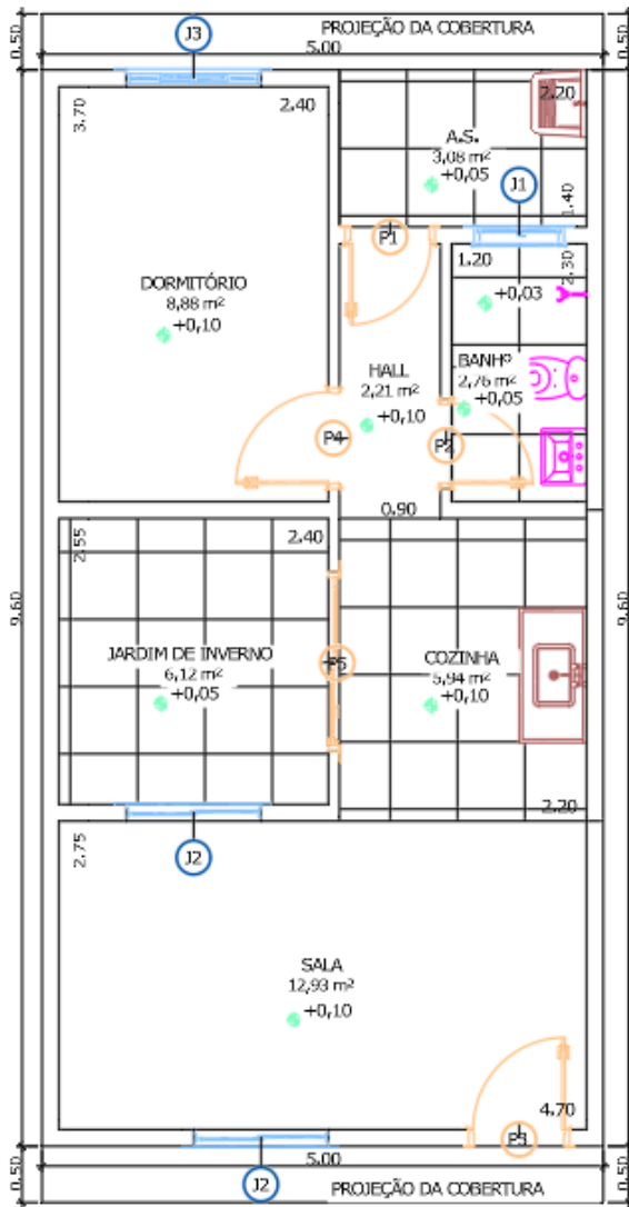
PLANTA BAIXA SEM ESCALA
