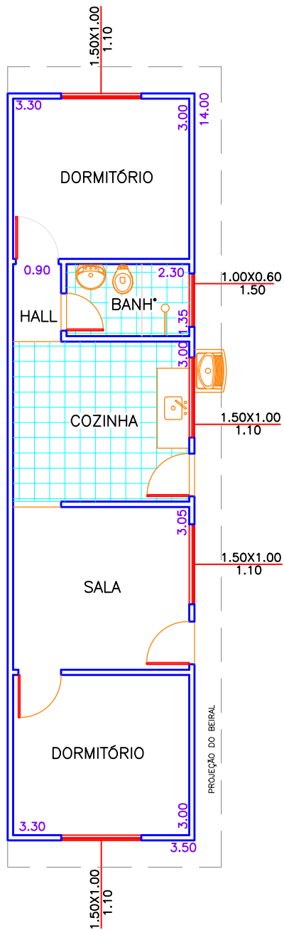
PLANTA BAIXA ESCALA 1:100
