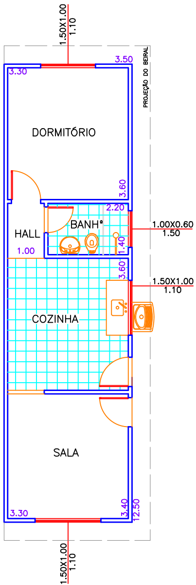
PLANTA BAIXA ESCALA 1:100
