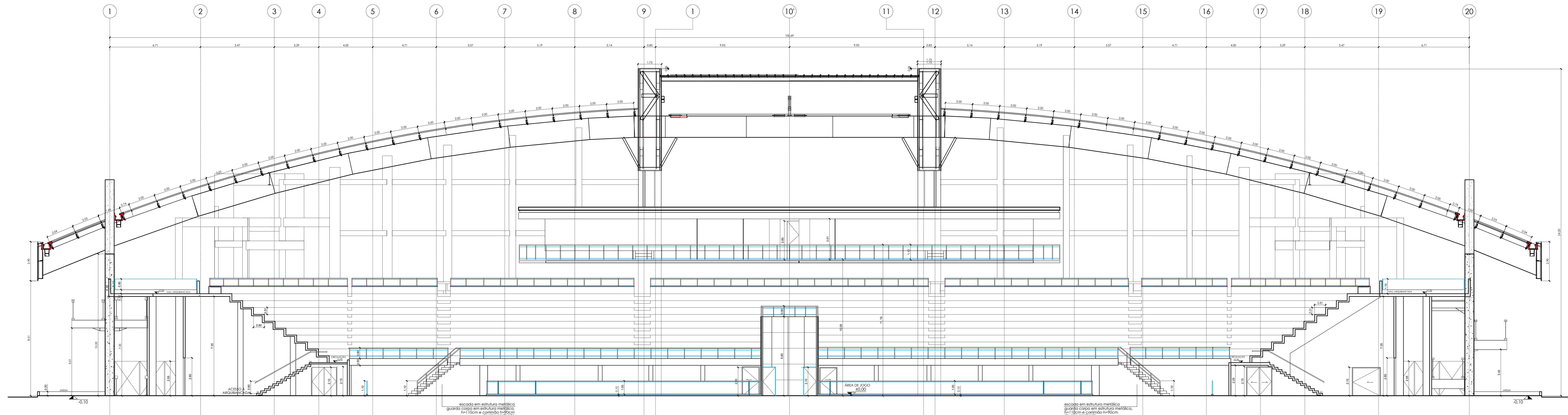
CORTE C-C ESCALA: 1/100
