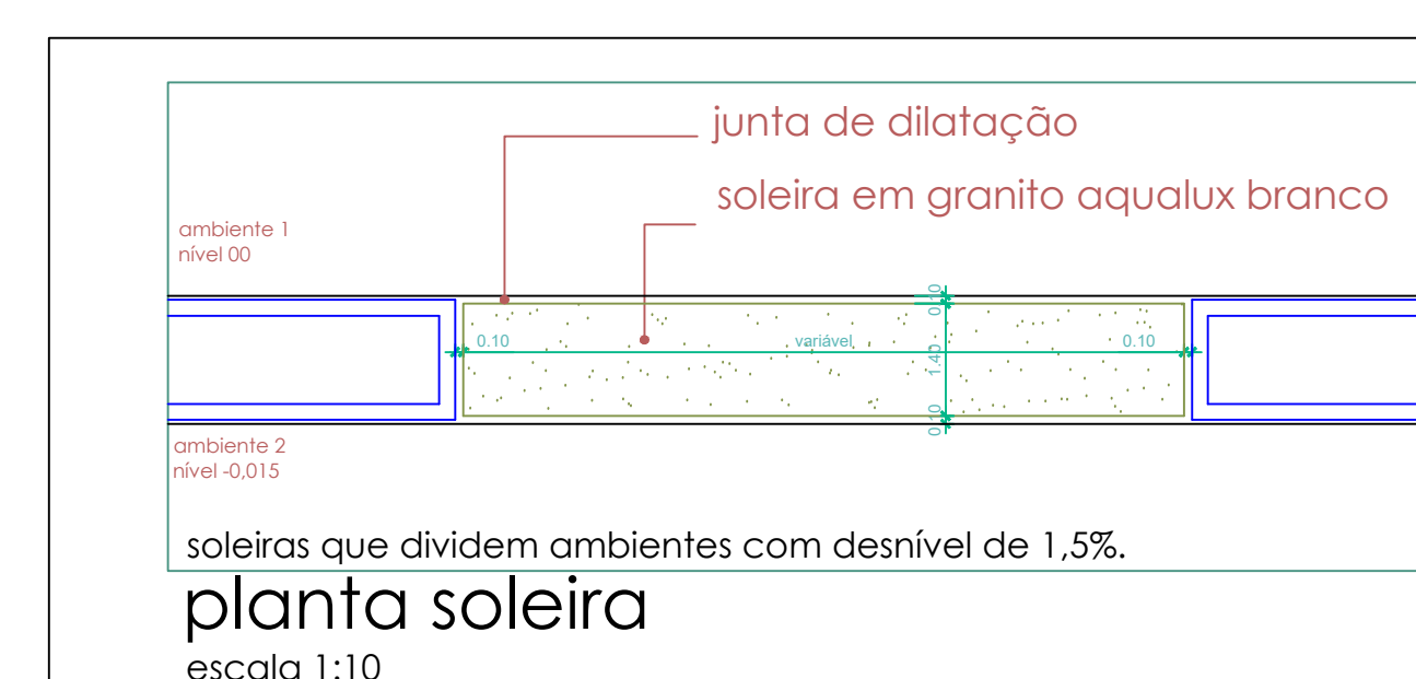
detalhe B
