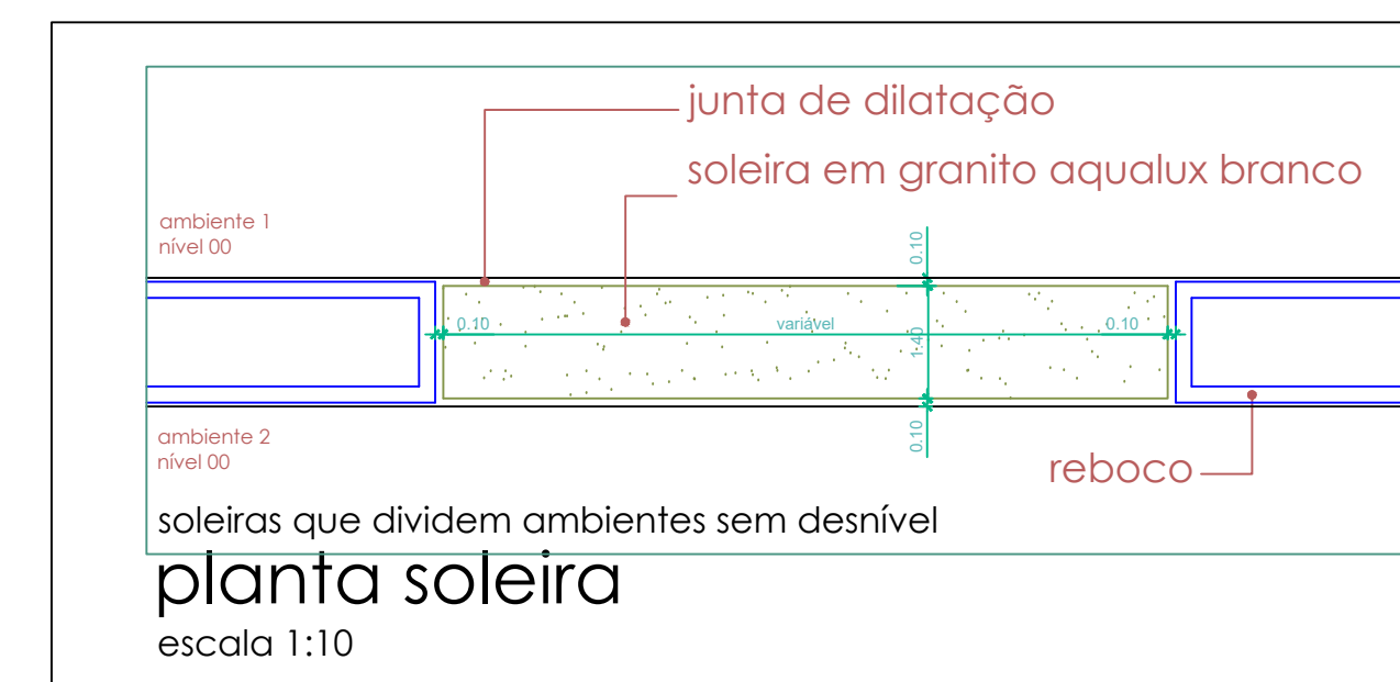
detalhe A
