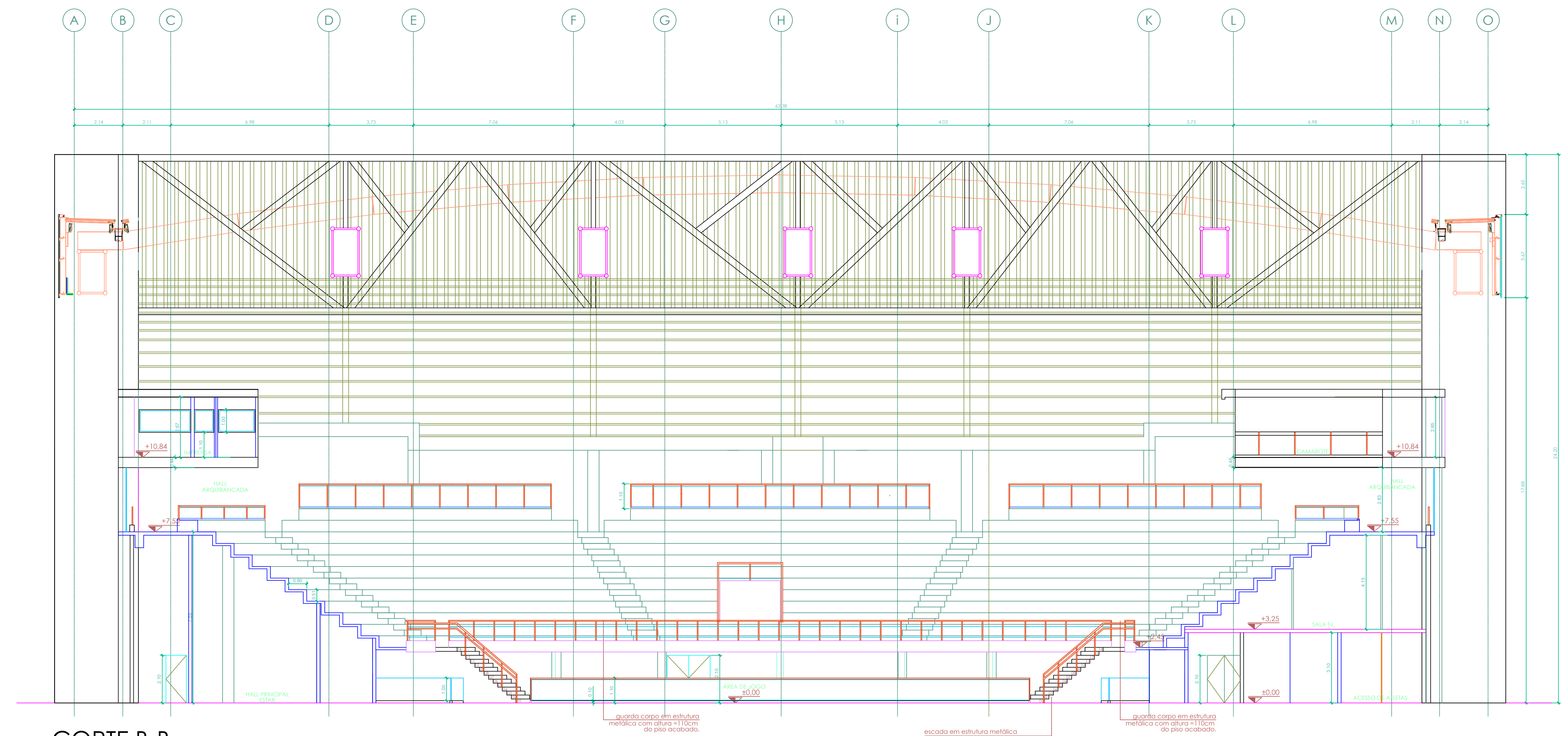
CORTE B-B ESCALA: 1/100
