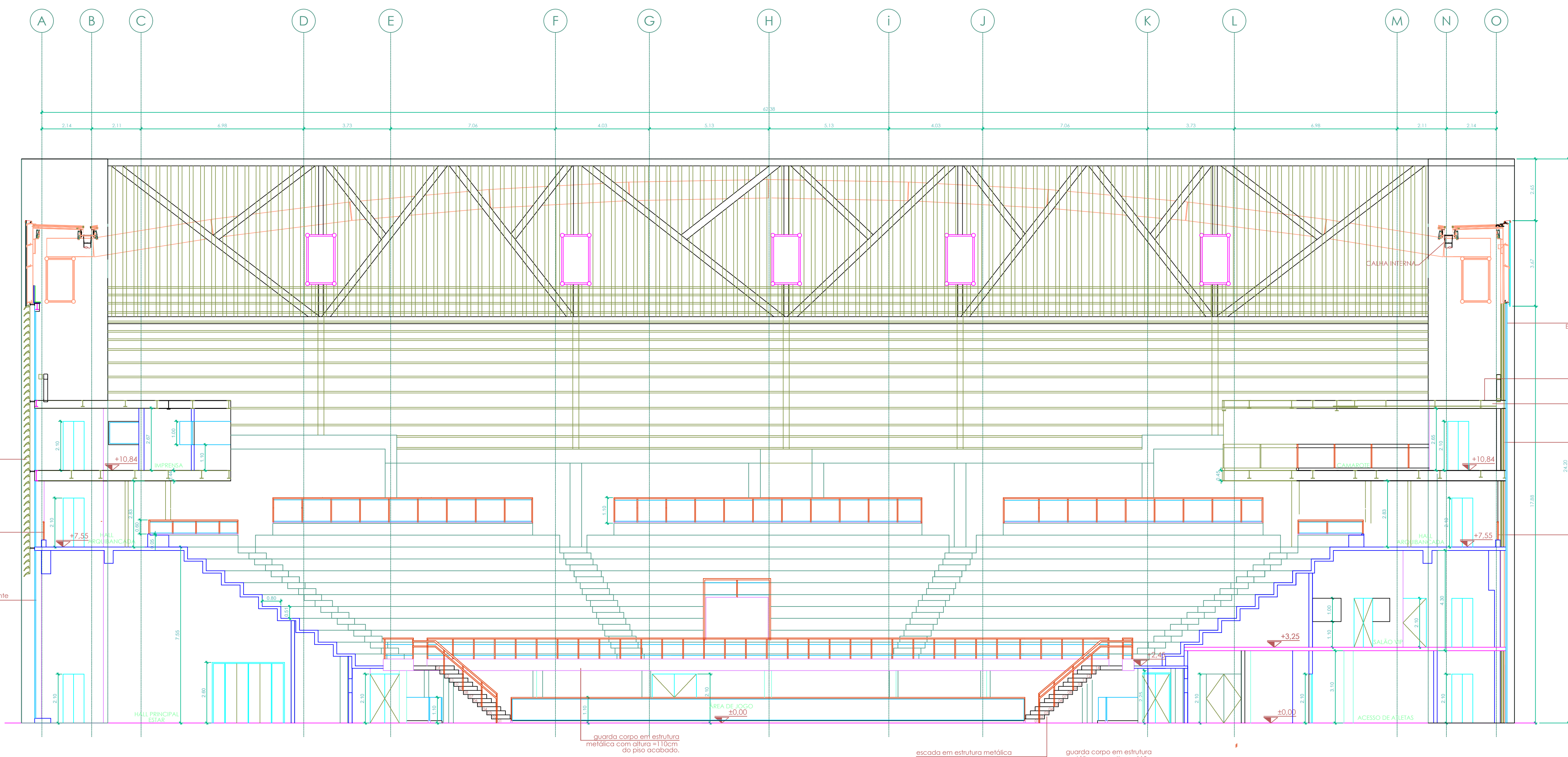
CORTE A-A ESCALA: 1/100
