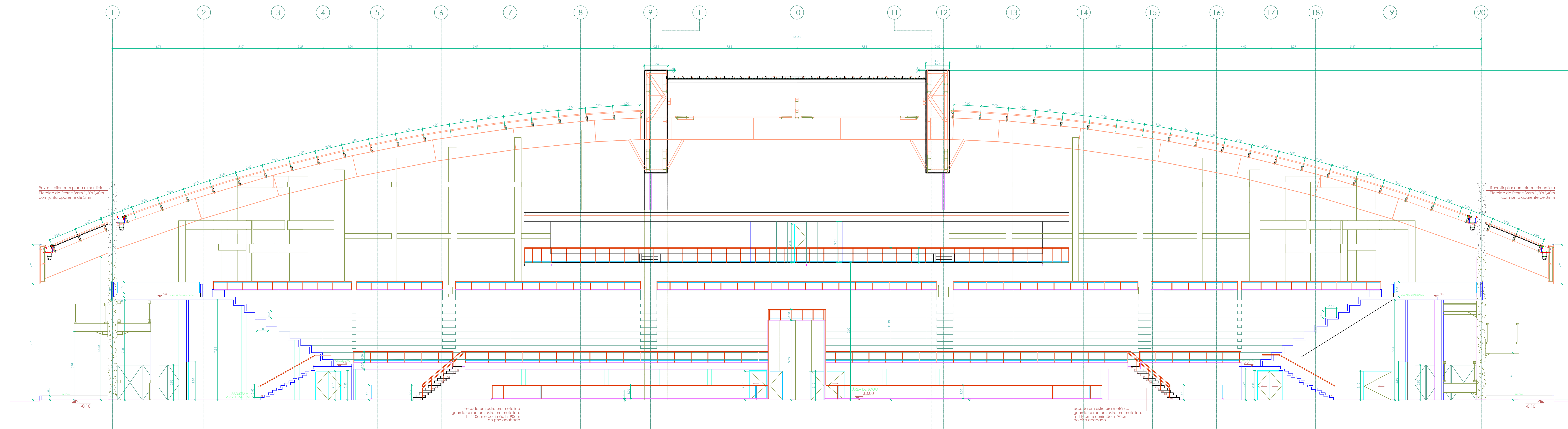
CORTE C-C ESCALA: 1/100
