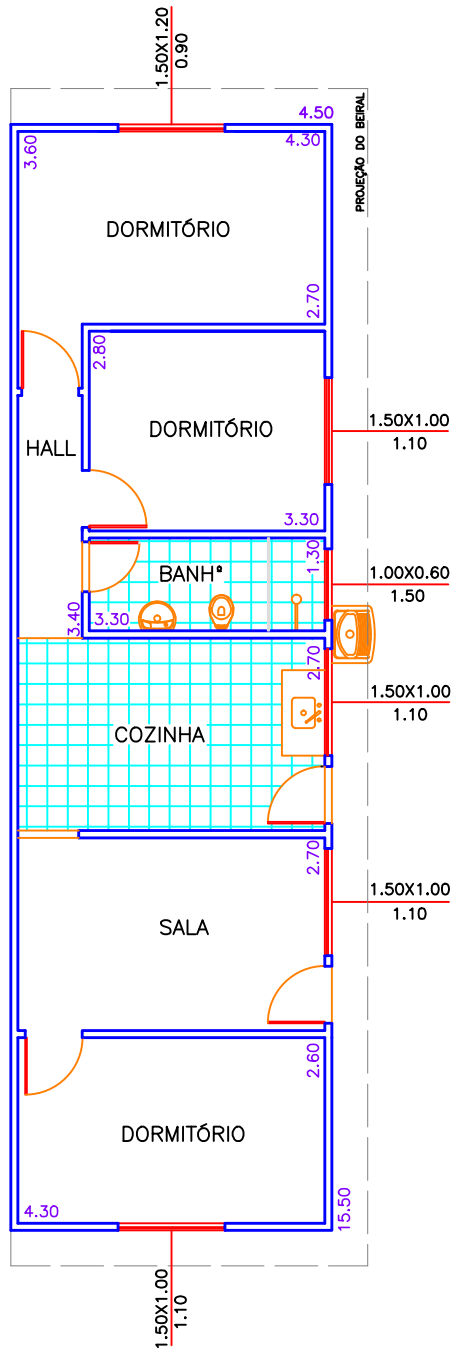
PLANTA BAIXA ESCALA 1:100
