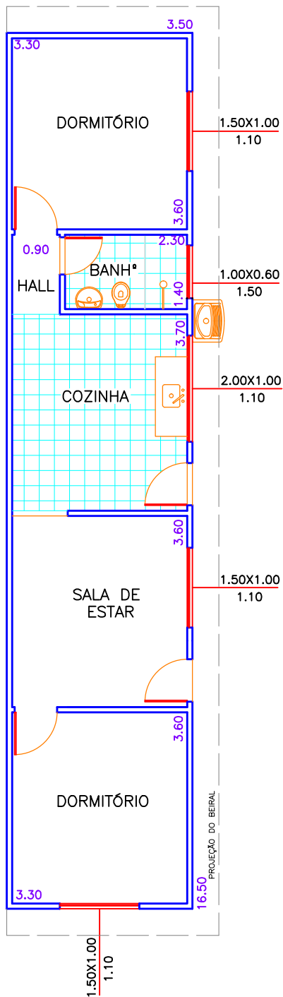
PLANTA BAIXA ESCALA 1:100
