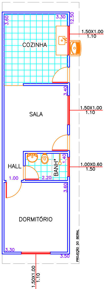
PLANTA BAIXA ESCALA 1:100
