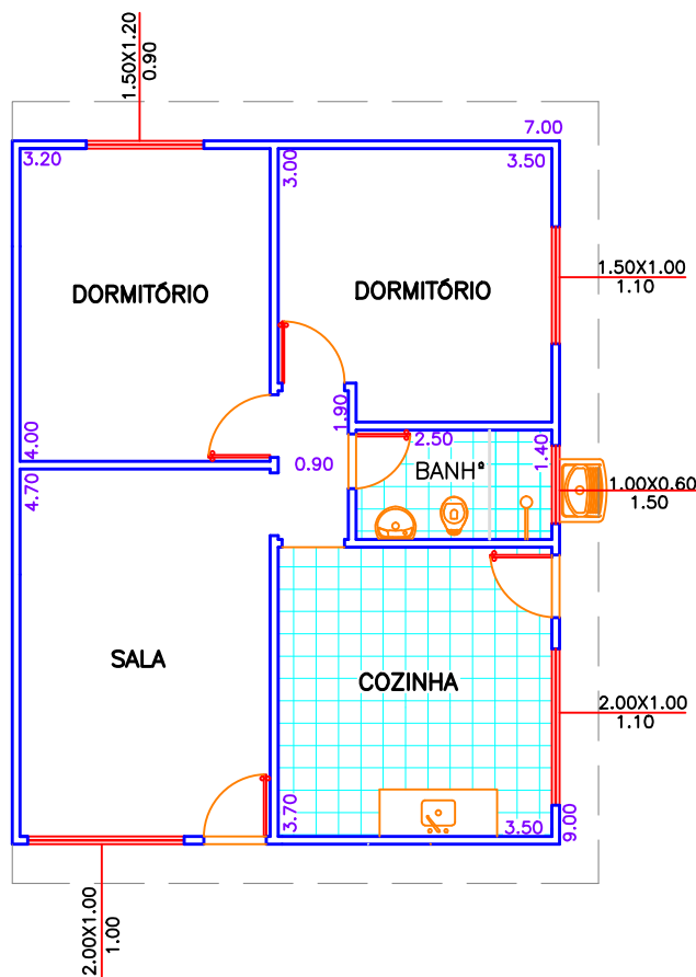
PLANTA BAIXA ESCALA 1:100
