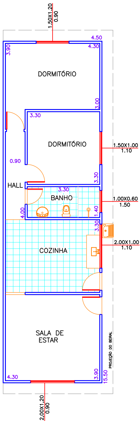
PLANTA BAIXA ESCALA 1:100
