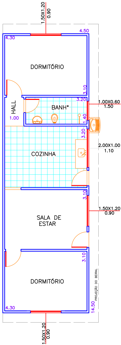
PLANTA BAIXA ESCALA 1:100
