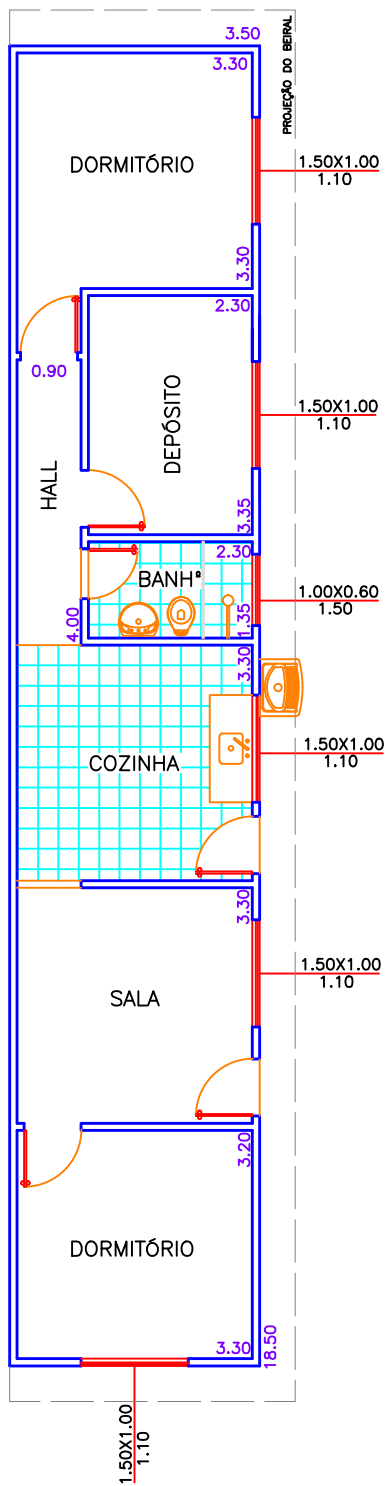
PLANTA BAIXA ESCALA 1:100
